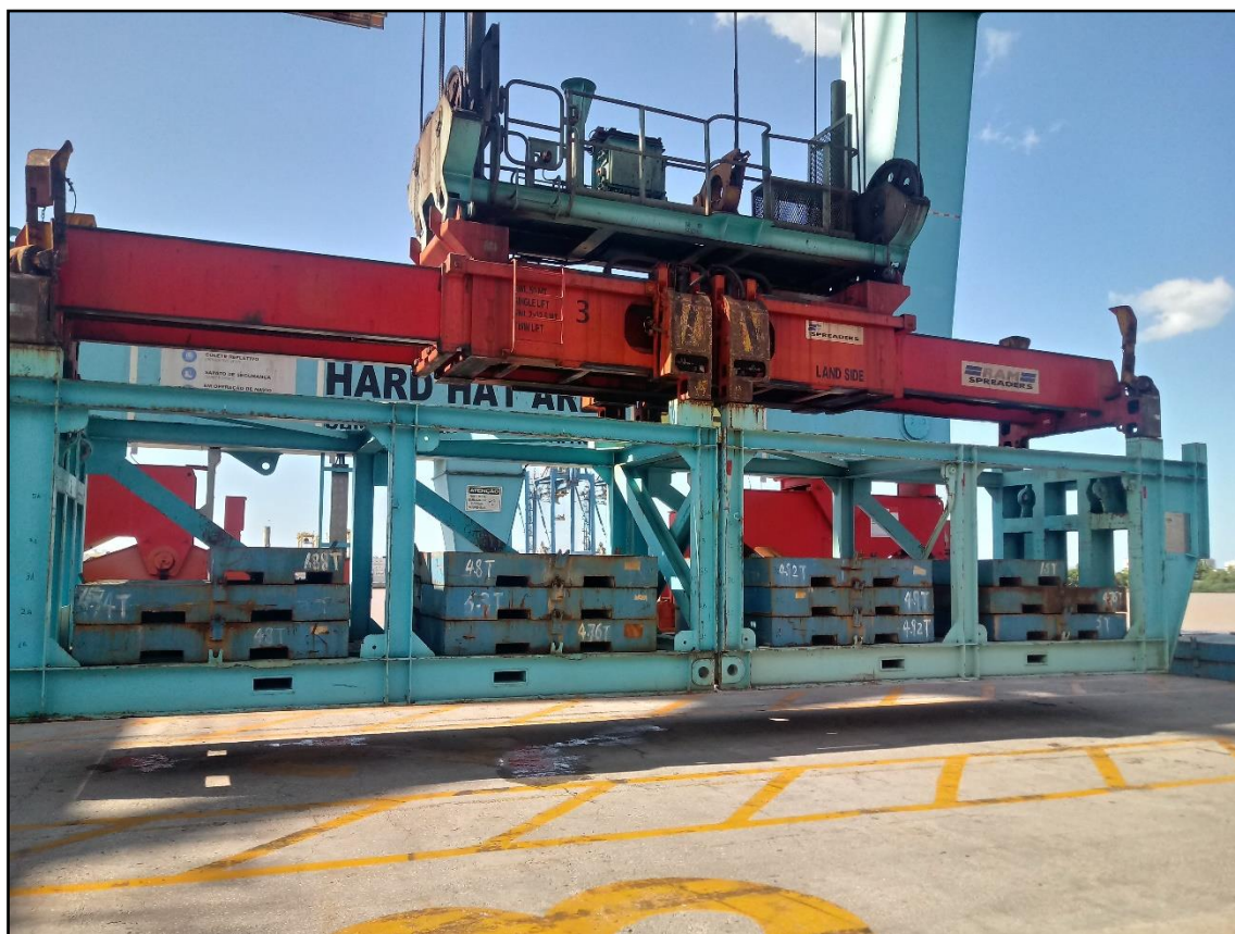
Figura 5. Teste de carga – Twin Lift.
