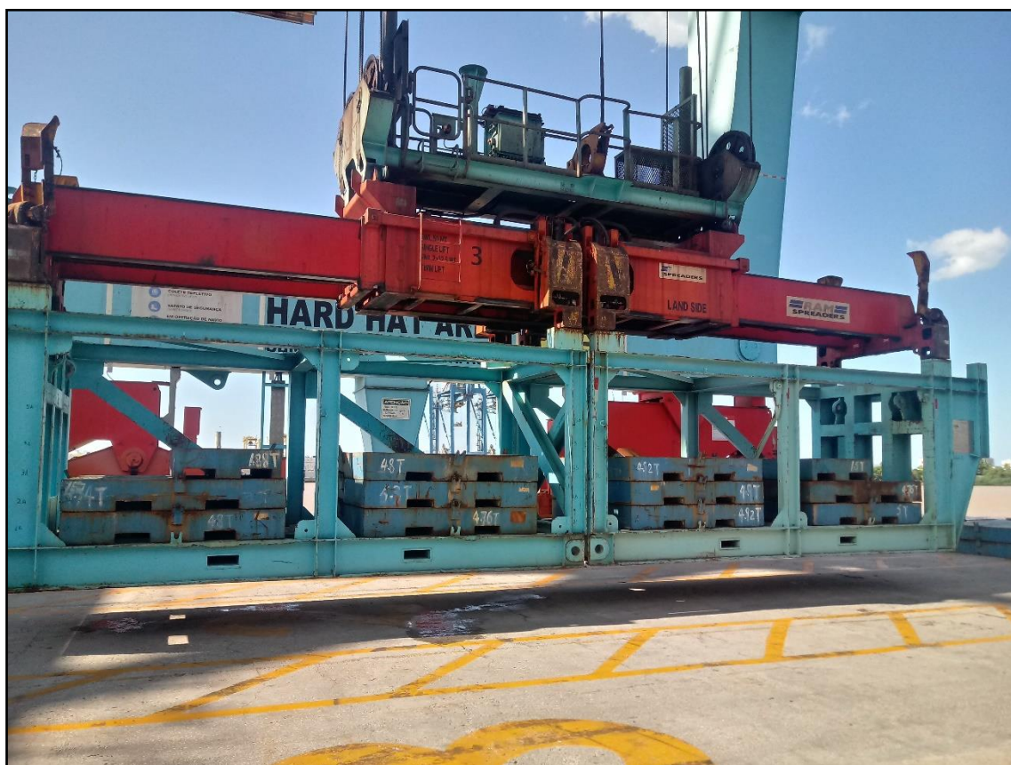
Figura 1. Spreader automático, SPR-03.
